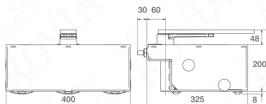
Rozměry pohonů BM5024
