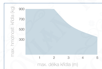
Limity použití BM5024
