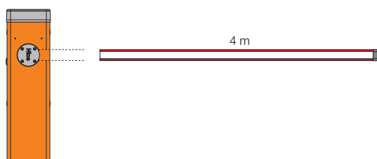
S4BAR dĺžka ramena 4 m Určené pre: ochranné gumené obloženie, smerové svetlá
