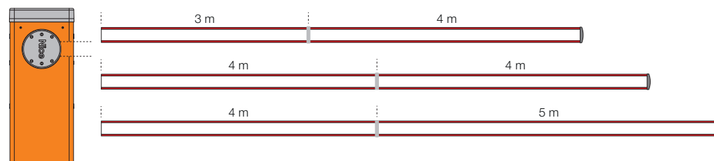
L9BAR Dĺžka ramena 7 m (3+4 m)* Určené pre: ochranné gumené obloženie, smerové svetlá, stojan (3 ks), mobilný stojan
