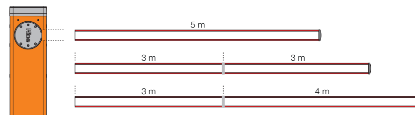
M7BAR Dĺžka ramena 5 m Určené pre: ochranné gumené obloženie, smerové svetlá, stojan (2 ks), mobilný stojan
