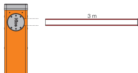
M3BAR Dĺžka ramena 3 m Určené pre: ochranné gumené obloženie, smerové svetlá
