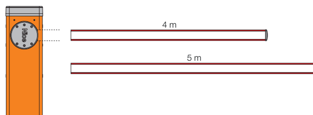
M5BAR Dĺžka ramena 4 m Určené pre: ochranné gumené obloženie, smerové svetlá, mobilný stojan
