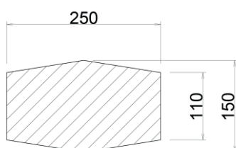
*Skúšobný hranol
