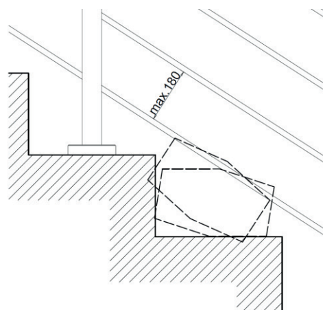
Cez žiadnu medzeru nesmie prejsť skúšobný hranol
