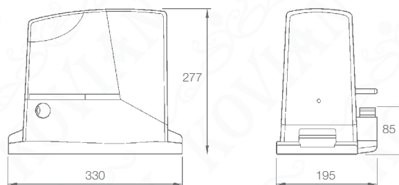
Rozměry pohonu RD400
