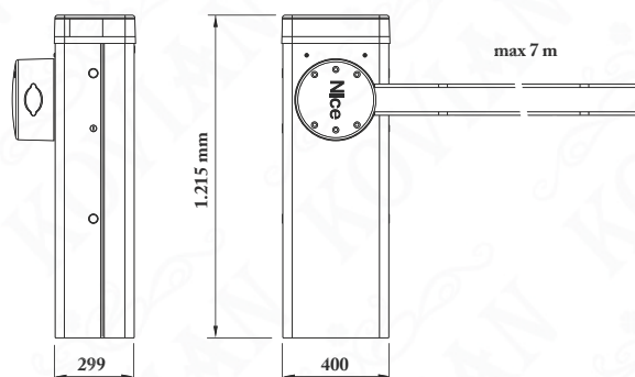
Rozměry závory M-BAR
